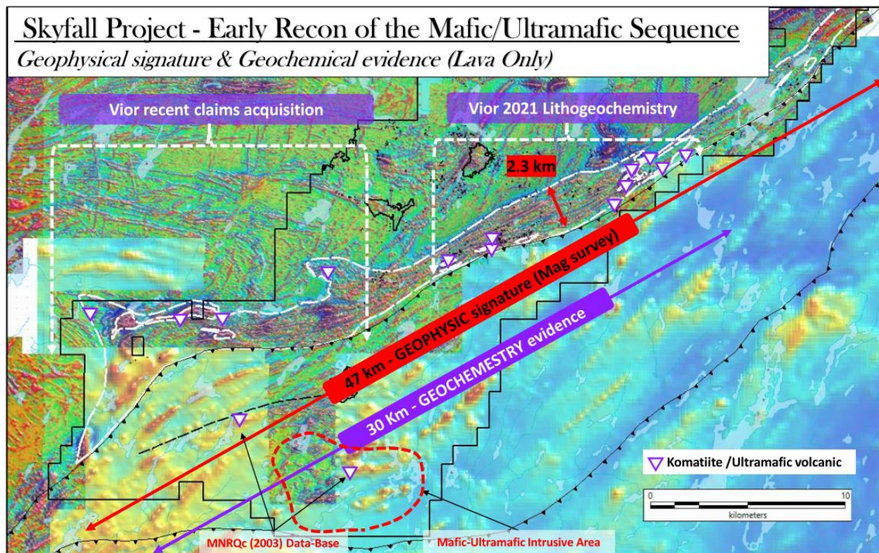
Figure 2: Séquence mafique/ultramafique
