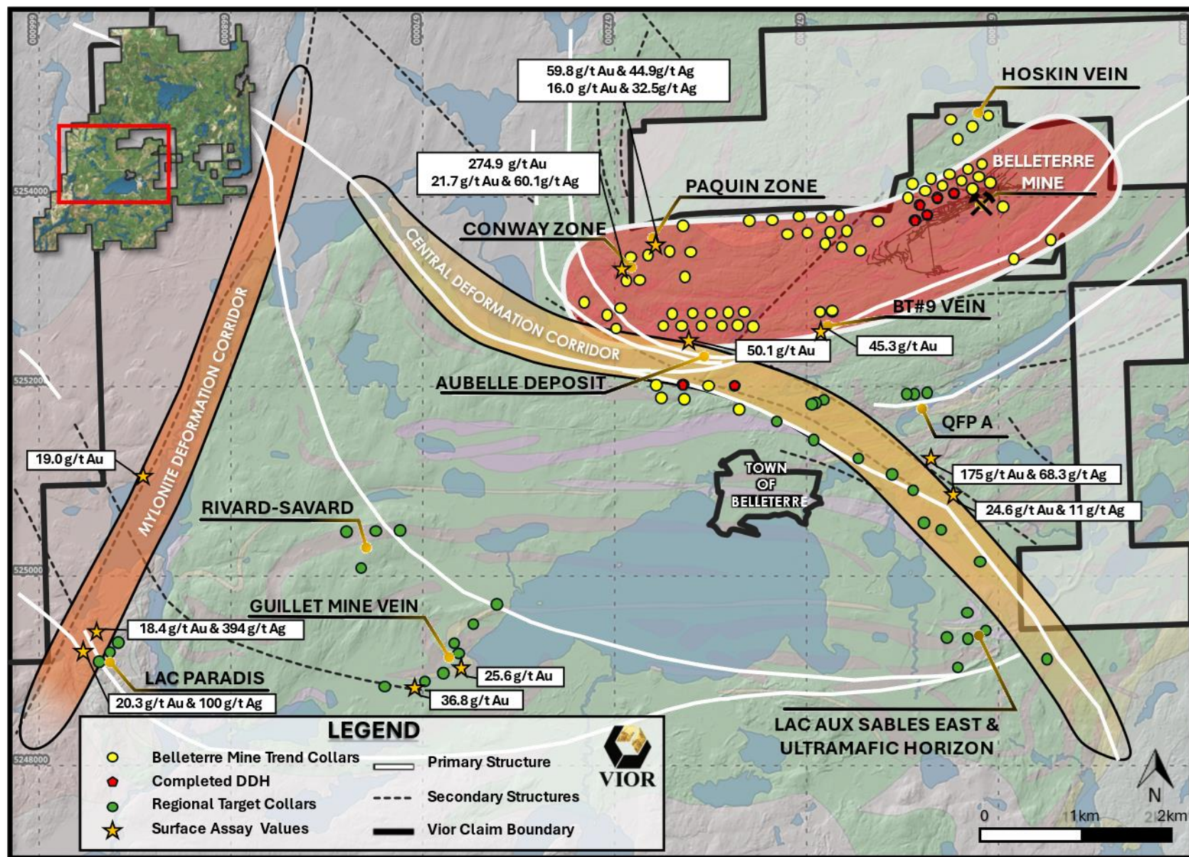
Figure 2: Localisation des cibles de forage, incluant celles complétées dans la séquence de la mine Belleterre
