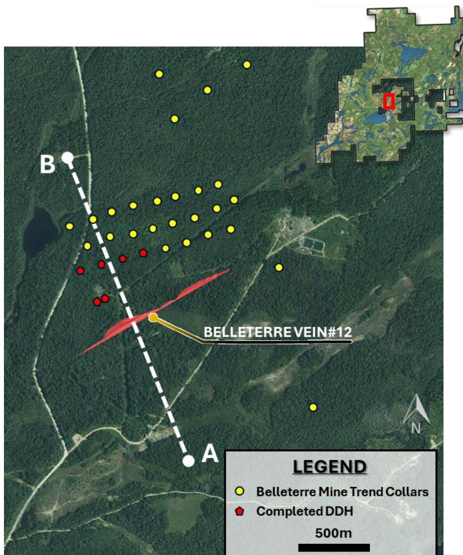
Figure 3: Site de la mine Belleterre – Localisation des cibles de forage
