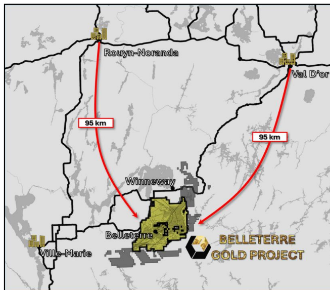
Figure 1: Localisation du projet Belleterre Or
