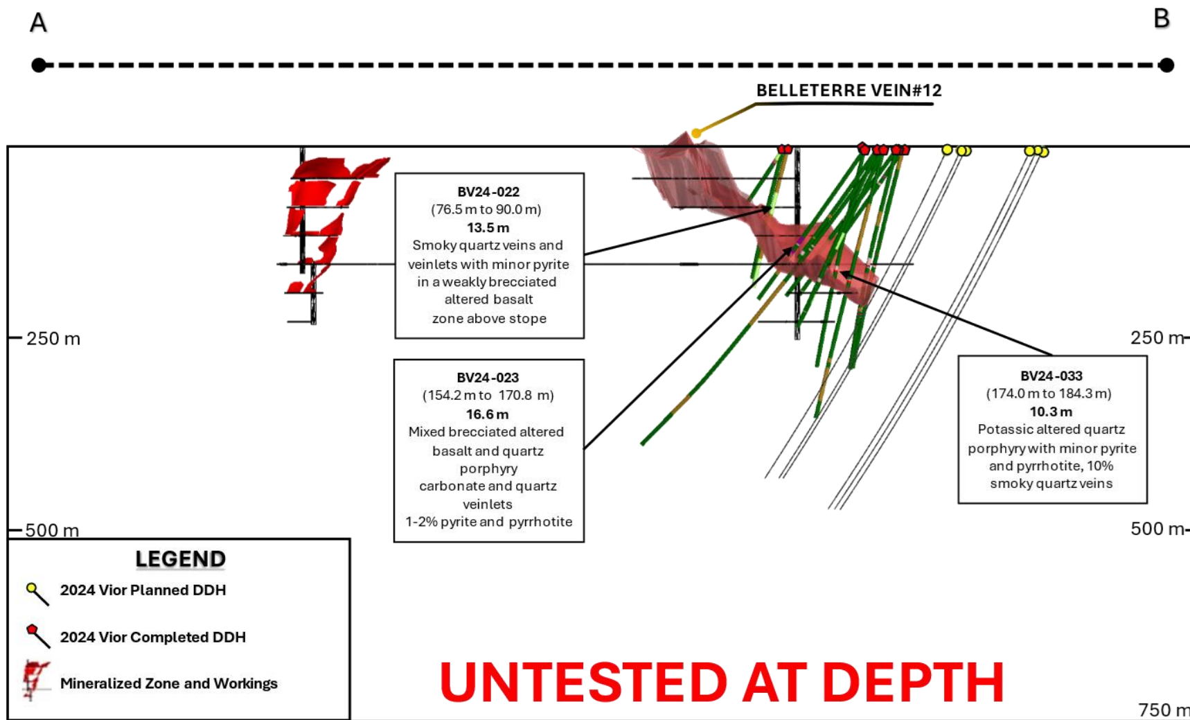
Figure 4: Mine Belleterre – Coupe transversal en direction de l'ouest, le long de la ligne A-B
